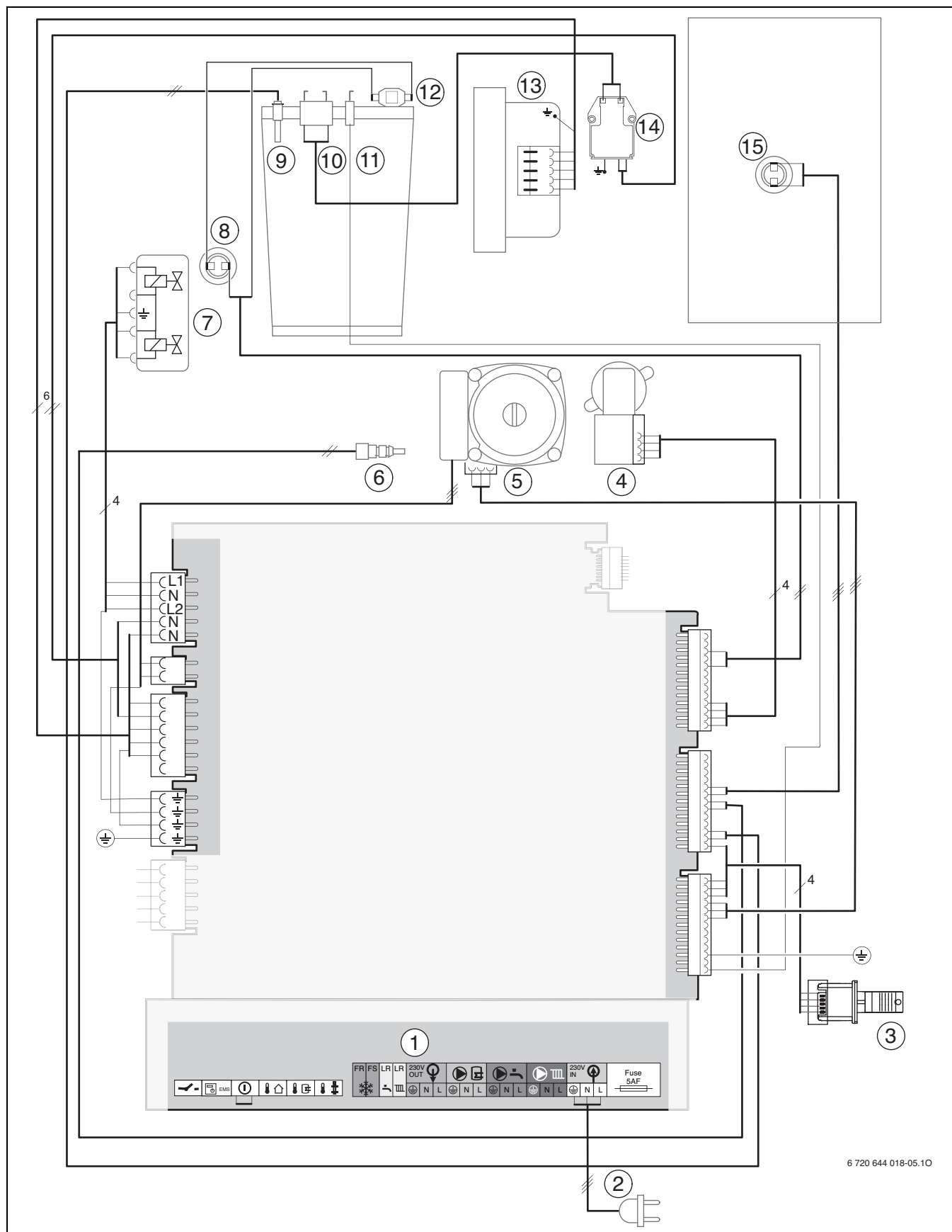
Мал. 72 Електромотаж
