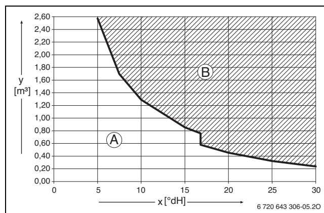
Мал. 16 Вимоги до води для заповнення та підживлення в °dH для приладів потужністю < 50 кВт
