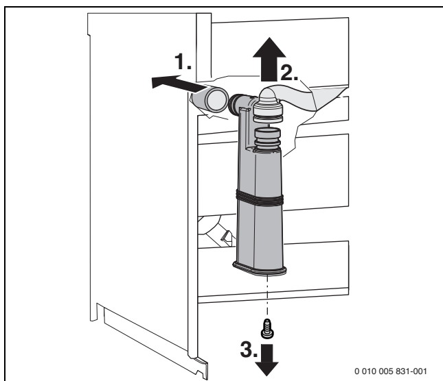
Σχ. 59 Αφαίρεση σιφονιού συμπυκνώματος
