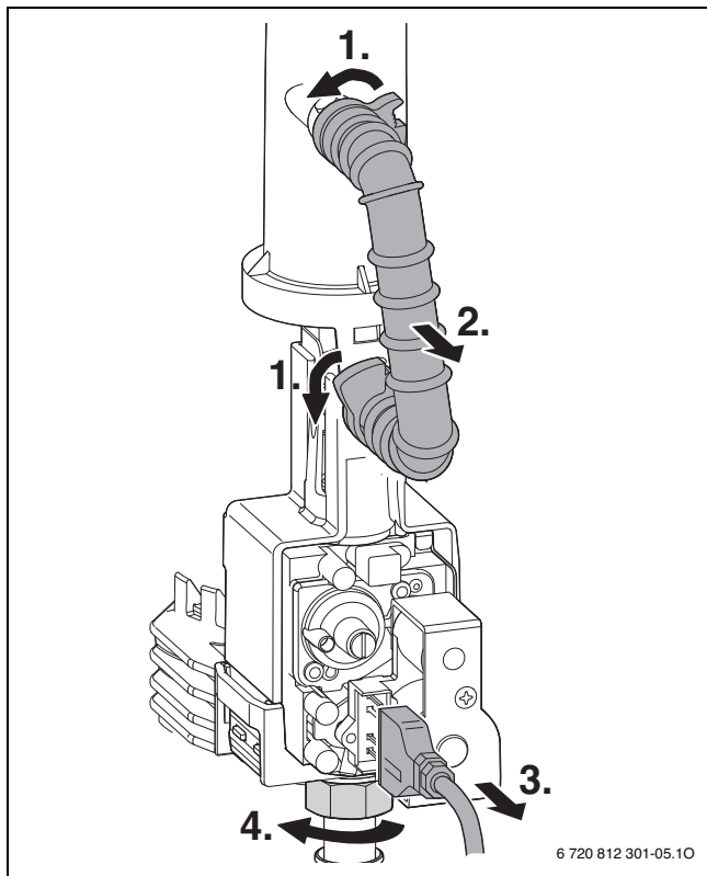
Σχ. 66 Αφαίρεση βάνας αερίου
