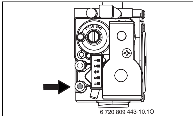
Σχ. 48 Στόμιο μέτρησης για πίεση σύνδεσης αερίου
