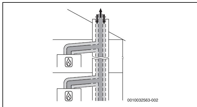
Σχ. 21 Πολλαπλή σύνδεση κατά C_{(10)3x} με ομόκεντρο αγωγό αέρα-καυσαερίων στον χώρο τοποθέτησης
