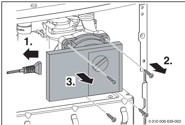
Σχ. 68 Αφαίρεση κυκλοφορητή θέρμανσης
