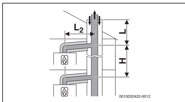
Σχ. 24 Πολλαπλή σύνδεση κατά C (14)3x με συλλογικό άκαμπτο αγωγό καυσαερίων και ομόκεντρο αγωγό αέρα-καυσαερίων στον χώρο εγκατάστασης
