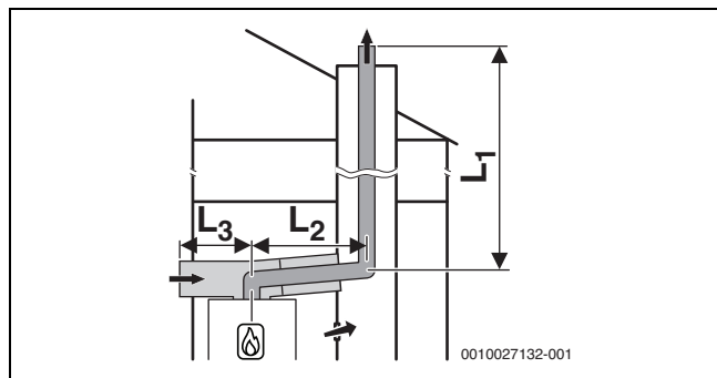
Σχ. 11 Άκαμπτος αγωγός καυσαερίων κατά C 53(x) στο φρεάτιο και αγωγός αέρα-καυσαερίων με ξεχωριστή παροχή αέρα και ομόκεντρη απαγωγή καυσαερίων στο χώρο εγκατάστασης
