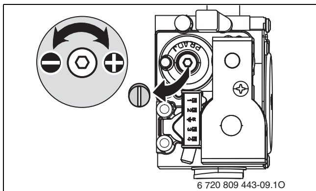
Σχ. 47 Αφαιρέστε τη σφράγιση από τη βίδα αερίου
