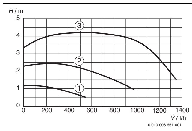
Σχ. 43 Χαρακτηριστική καμπύλη του κυκλοφορητή θέρμανσης (προσαρμοσμένη ταχύτητα)
