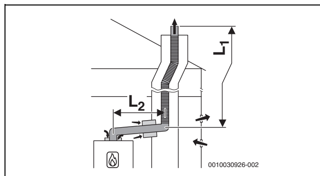
Σχ. 19 Εύκαμπτος αγωγός καυσαερίων κατά B 23p /B 53p με παροχή αέρα από τον χώρο εγκατάστασης στη συσκευή και ομόκεντρο στοιχείο σύνδεσης ανάμεσα στον χώρο εγκατάστασης και το φρεάτιο
