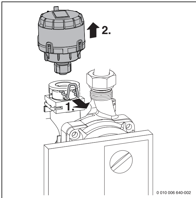
Σχ. 69 Αφαίρεση κινητήρα της τριόδου βάνας
