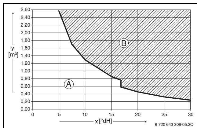
Σχ. 28 Απαιτήσεις για το νερό πλήρωσης και συμπλήρωσης σε °dH για συσκευές < 50 kW
