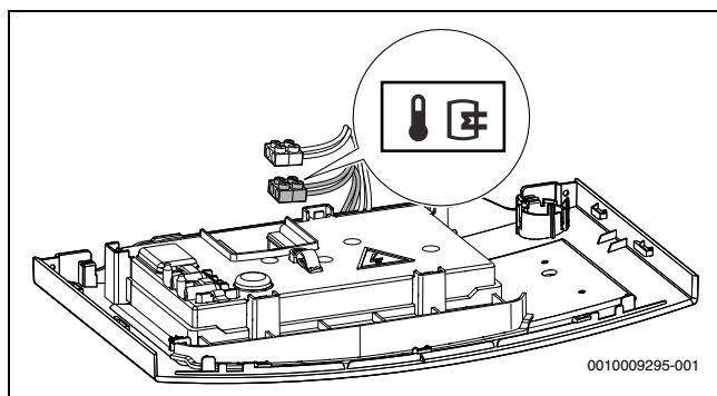
Σχ. 39 Σύνδεση αισθητήρα θερμοκρασίας μπόιλερ
