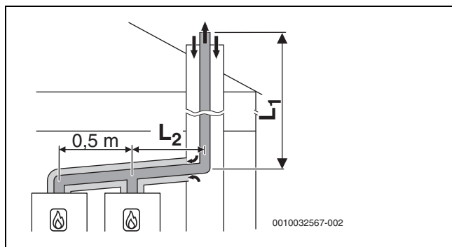
Σχ. 27 Συστοιχία μονάδων με 2 συσκευές: Άκαμπτος αγωγός καυσαερίων κατά C 93x στο φρεάτιο και ομόκεντρος αγωγός αέρα-καυσαερίων στον χώρο εγκατάστασης
