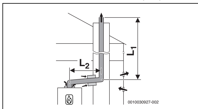
Σχ. 18 Άκαμπτος αγωγός καυσαερίων κατά B 23p /B 53p με παροχή αέρα από τον χώρο εγκατάστασης στη συσκευή και ομόκεντρο στοιχείο σύνδεσης ανάμεσα στον χώρο εγκατάστασης και το φρεάτιο
