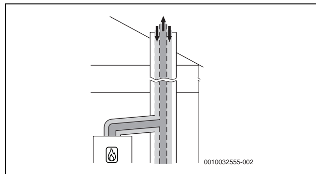
Σχ. 10 Ομόκεντρος αγωγός αέρα-καυσαερίων κατά C 43(x) στον χώρο τοποθέτησης
