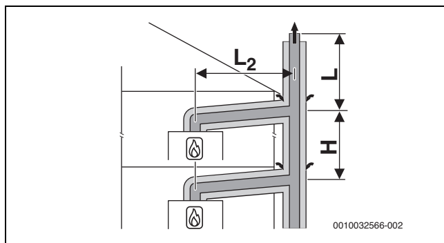
Σχ. 23 Πολλαπλή σύνδεση κατά C_{(13)3x} με ομόκεντρο αγωγό αέρα-καυσαερίων στον εξωτερικό τοίχο και στον χώρο εγκατάστασης
