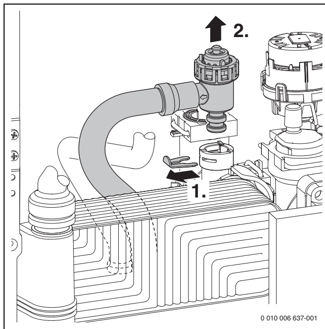
Σχ. 61 Αφαίρεση βαλβίδας ασφαλείας (κύκλωμα θέρμανσης)
