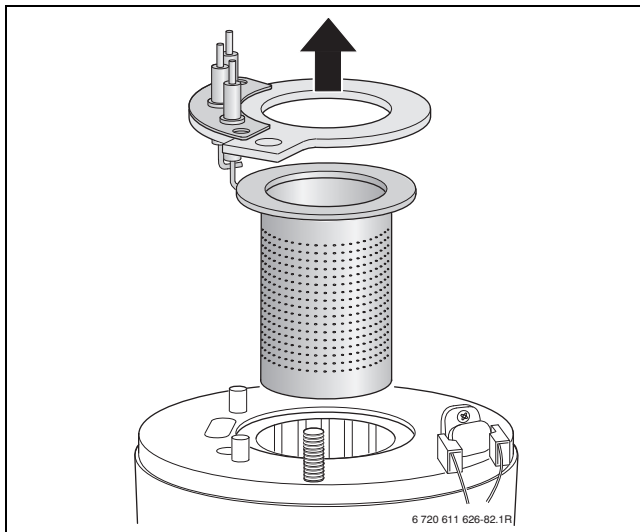
Σχ. 53 Αφαίρεση καυστήρα
