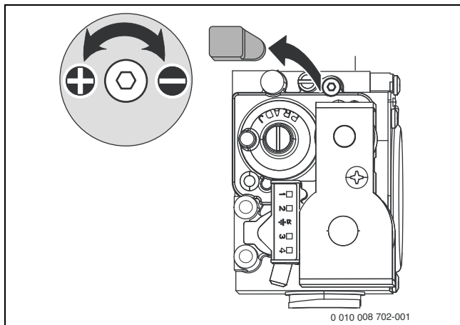
Σχ. 46 Αφαιρέστε τη σφράγιση
