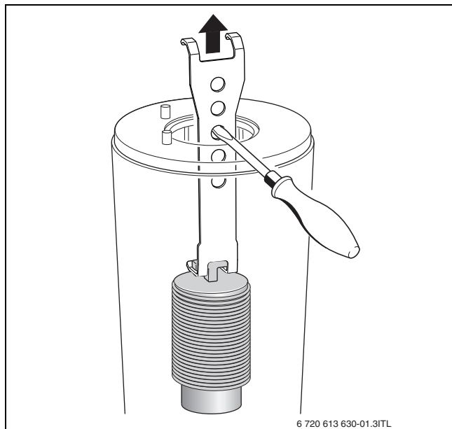
Σχ. 55 Αφαίρεση κάτω μετατοπιζόμενου σώματος
