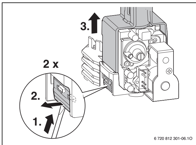
Σχ. 67 Αφαίρεση βάνας αερίου
