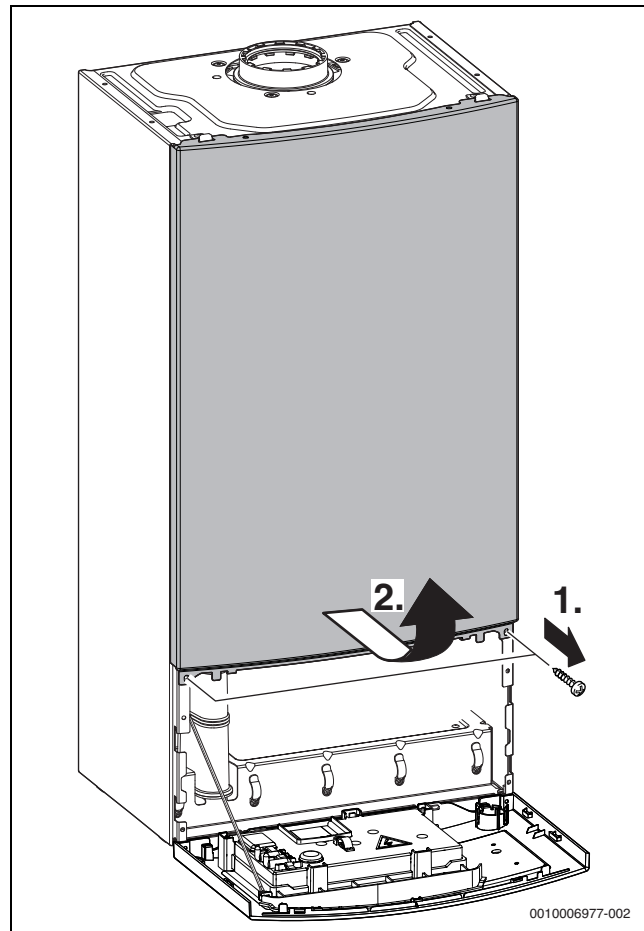
Σχ. 33 Αφαίρεση μπροστινού καλύμματος
