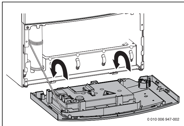
Σχ. 32 Μετακίνηση μονάδας ελέγχου σε θέση Service
