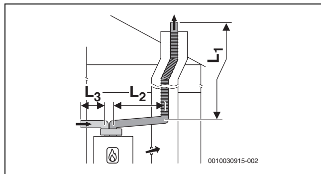
Σχ. 14 Εύκαμπτος αγωγός καυσαερίων κατά C 53 στο φρεάτιο και αγωγός αέρα-καυσαερίων με ξεχωριστούς σωλήνες για παροχή αέρα και απαγωγή καυσαερίων στον χώρο εγκατάστασης
