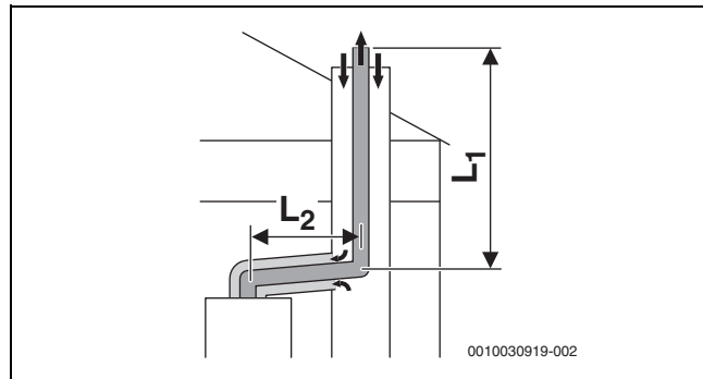
Σχ. 16 Άκαμπτος αγωγός καυσαερίων κατά C 93x στο φρεάτιο και ομόκεντρος αγωγός αέρα-καυσαερίων στον χώρο εγκατάστασης
