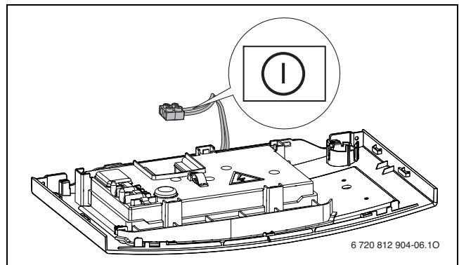
Σχ. 38 Εξωτερική επαφή μεταγωγής, ελεύθερου δυναμικού
