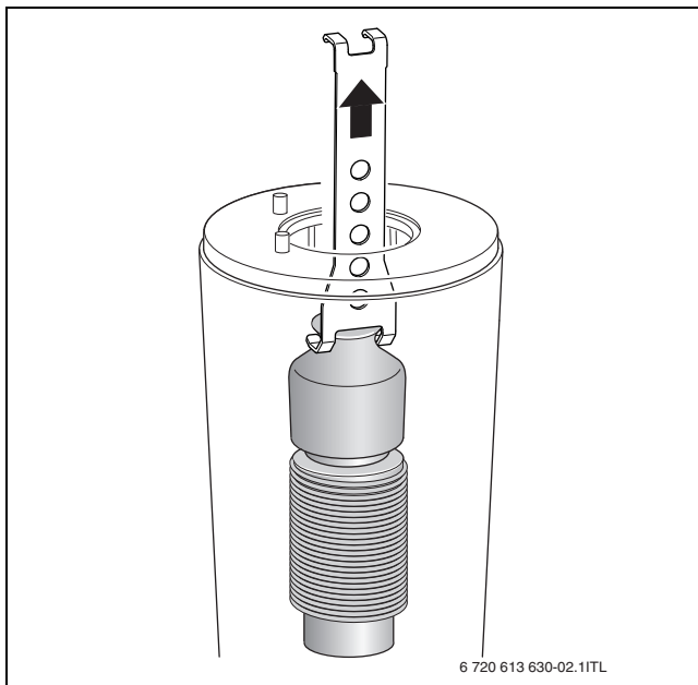
Σχ. 54 Αφαίρεση επάνω μετατοπιζόμενου σώματος
