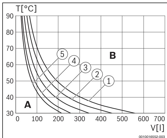
Σχ. 30 Χαρακτηριστικές καμπύλες του δοχείου διαστολής
