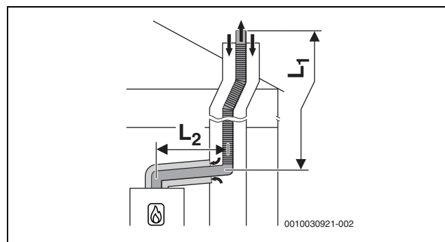
Σχ. 17 Εύκαμπτος αγωγός καυσαερίων κατά C 93x στο φρεάτιο και ομόκεντρος αγωγός αέρα-καυσαερίων στον χώρο εγκατάστασης
