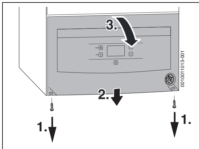
Σχ. 31 Αναδίπλωση μονάδας ελέγχου προς τα κάτω
