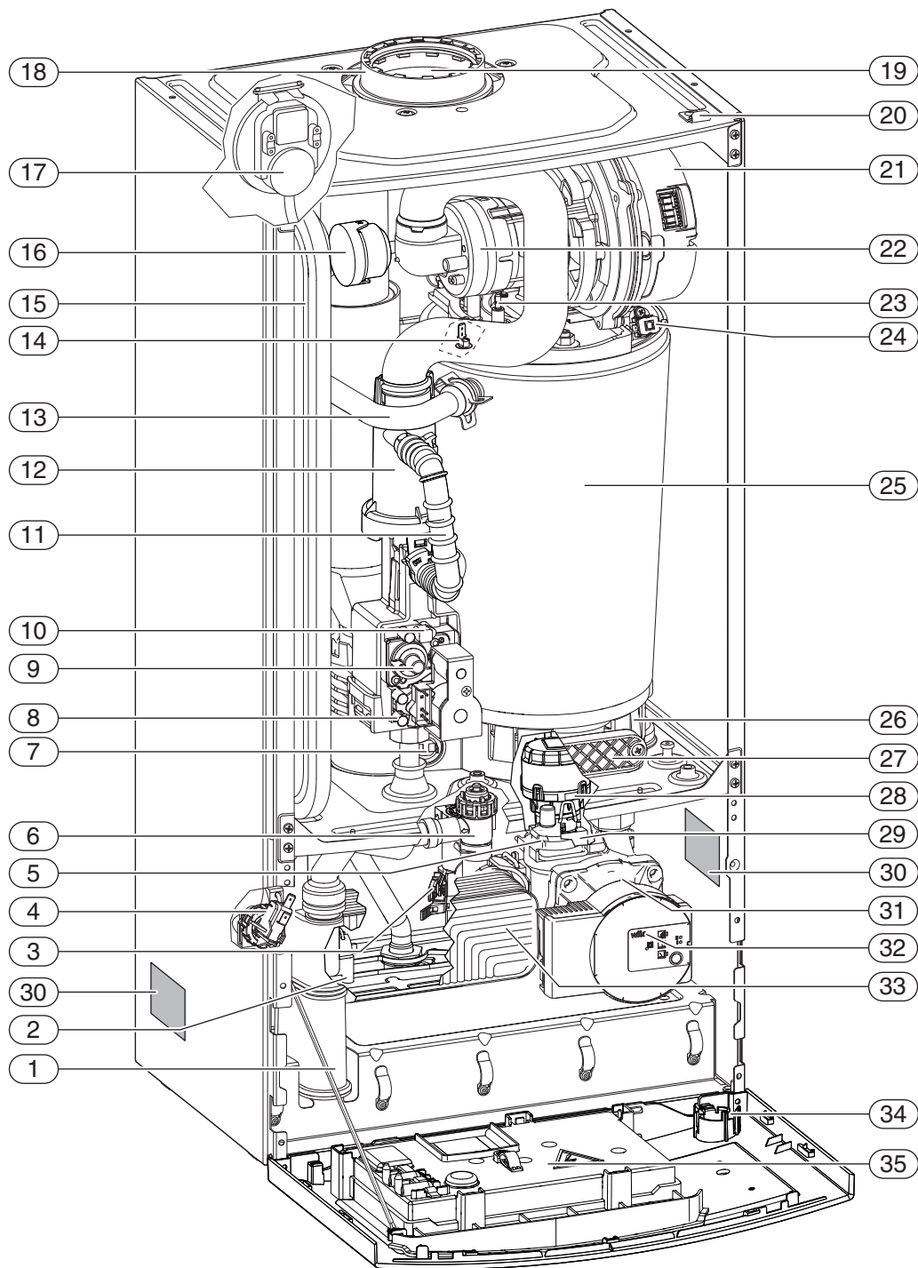
Σχ. 3 Επισκόπηση του προϊόντος
