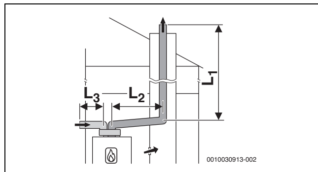
Σχ. 13 Άκαμπτος αγωγός καυσαερίων κατά C 53 στο φρεάτιο και αγωγός αέρα-καυσαερίων με ξεχωριστούς σωλήνες για παροχή αέρα και απαγωγή καυσαερίων στο χώρο εγκατάστασης
