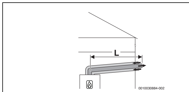
Σχ. 6 Οριζόντιος ομόκεντρος αγωγός αέρα-καυσαερίων κατά C 13x μέσω του εξωτερικού τοίχου
