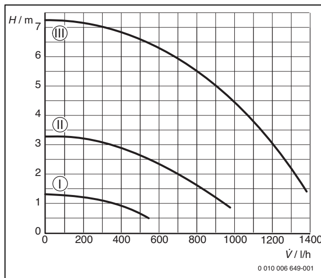
Σχ. 42 Χαρακτηριστική καμπύλη του κυκλοφορητή θέρμανσης (σταθερή ταχύτητα)
