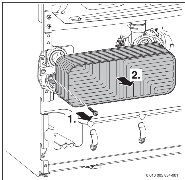
Σχ. 63 Αφαίρεση πλακοειδούς εναλλάκτη θερμότητας
