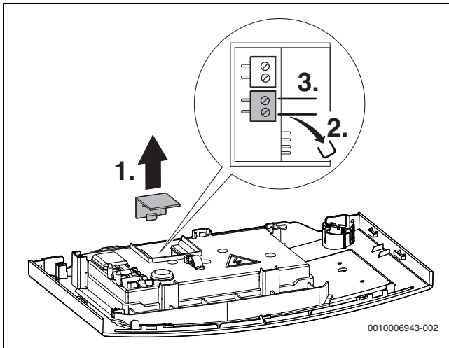
Σχ. 35 Σύνδεση θερμοστάτη
