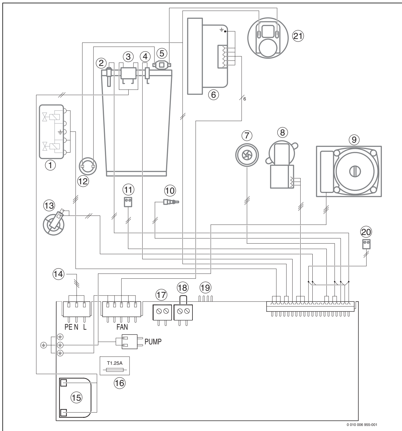
Σχ. 72 Ηλεκτρική καλωδίωση
