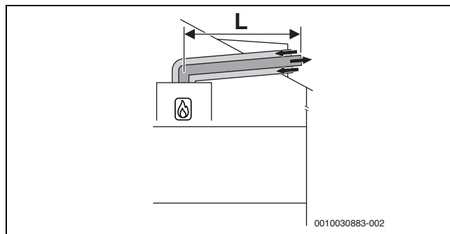
Σχ. 7 Οριζόντιος ομόκεντρος αγωγός αέρα-καυσαερίων κατά C 13x μέσω της στέγης
