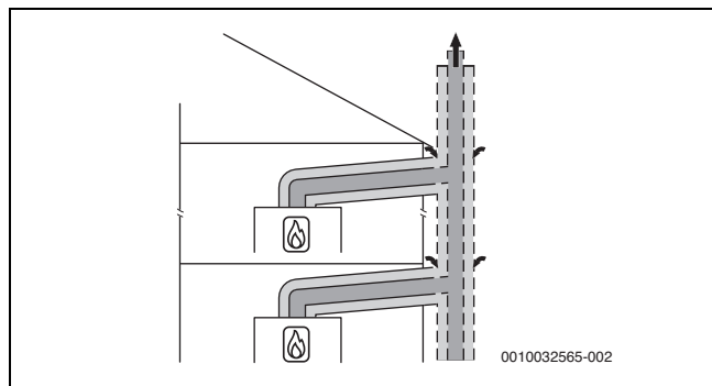
Σχ. 22 Πολλαπλή σύνδεση κατά C_{(12)3x} με ομόκεντρο αγωγό αέρα-καυσαερίων στον χώρο εγκατάστασης
