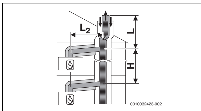
Σχ. 25 Πολλαπλή σύνδεση κατά C (14)3x με συλλογικό εύκαμπτο αγωγό απαγωγής καυσαερίων και ομόκεντρο αγωγό αέρα-καυσαερίων στον χώρο εγκατάστασης
