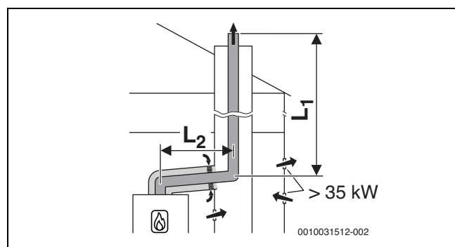
Σχ. 20 Άκαμπτος αγωγός καυσαερίων στο φρεάτιο κατά B 33 με παροχή αέρα από τον χώρο εγκατάστασης μέσω του ομόκεντρου αγωγού αέρα-καυσαερίων στον χώρο εγκατάστασης
