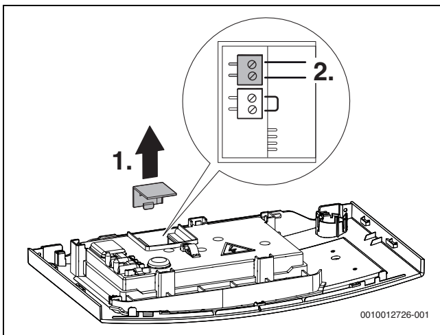
Σχ. 36 Σύνδεση αισθητήρα εξωτερικής θερμοκρασίας
