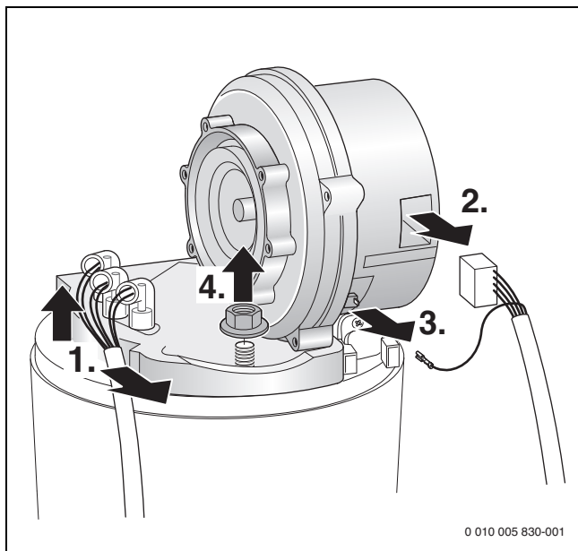
Σχ. 52 Αφαίρεση ανεμιστήρα
