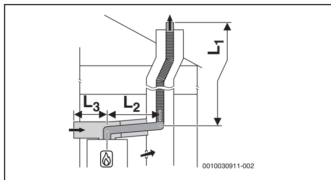
Σχ. 12 Εύκαμπτος αγωγός καυσαερίων κατά C 53(x) στο φρεάτιο και αγωγός αέρα-καυσαερίων με ξεχωριστή παροχή αέρα και ομόκεντρη απαγωγή καυσαερίων στο χώρο εγκατάστασης
