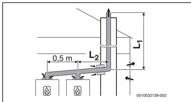
Σχ. 26 Συστοιχία μονάδων με 2 συσκευές: Άκαμπτος αγωγός καυσαερίων στο φρεάτιο κατά B 23p /B 53p με παροχή αέρα από τον χώρο εγκατάστασης στη συσκευή
