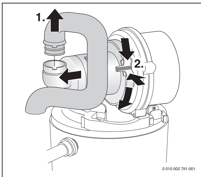
Σχ. 51 Αφαίρεση σωλήνα αναρρόφησης και διάταξης ανάμειξης
