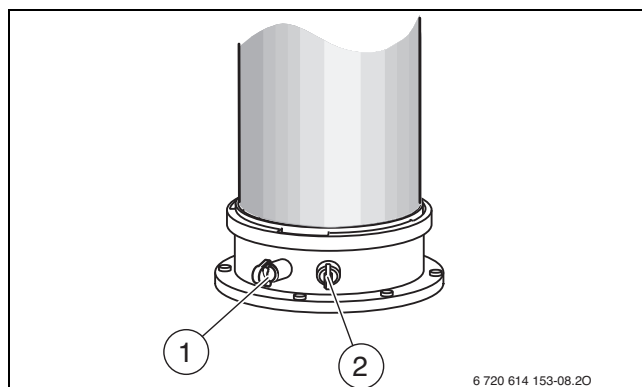
Σχ. 49 Στόμιο μέτρησης καυσαερίων και στόμιο μέτρησης αέρα καύσης
