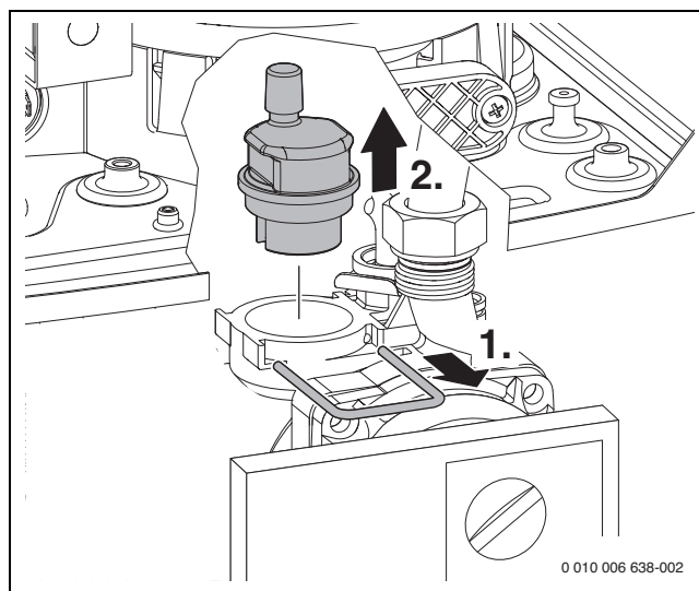
Σχ. 64 Αφαίρεση αυτόματου εξαεριστήρα
