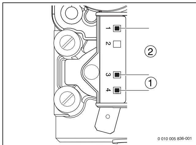
Σχ. 65 Σημεία μέτρησης στη βάνα αερίου
