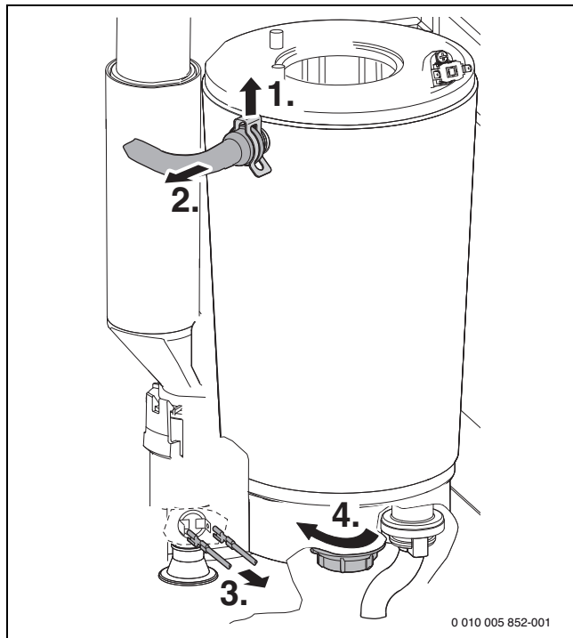
Σχ. 70 Λύσιμο σωλήνα προσαγωγής και αποσύνδεση καλωδίου
