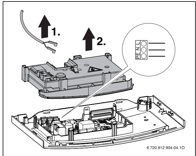
Σχ. 37 Αντικατάσταση καλωδίου τροφοδοσίας
