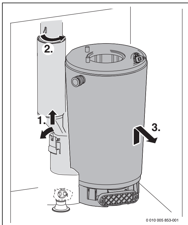
Σχ. 71 Αφαίρεση εναλλάκτη θερμότητας
