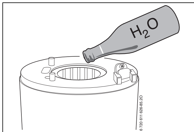
Σχ. 58 Έκπλυση εναλλάκτη θερμότητας με νερό
