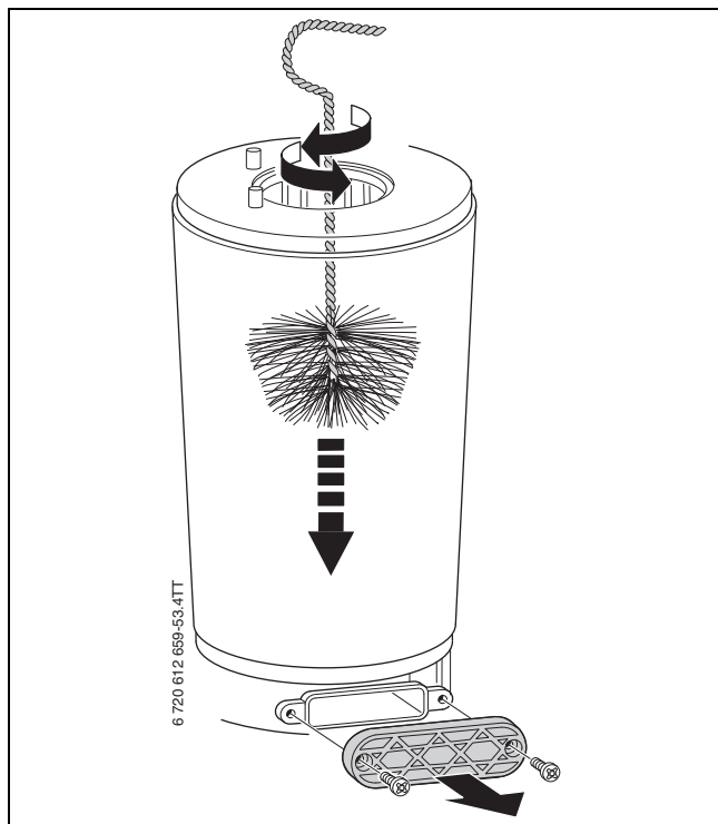
Σχ. 56 Καθαρισμός εναλλάκτη
