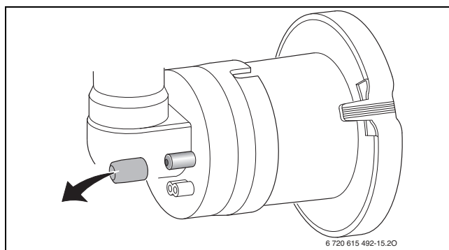
Σχ. 50 Στόμιο μέτρησης στη διάταξη ανάμειξης
