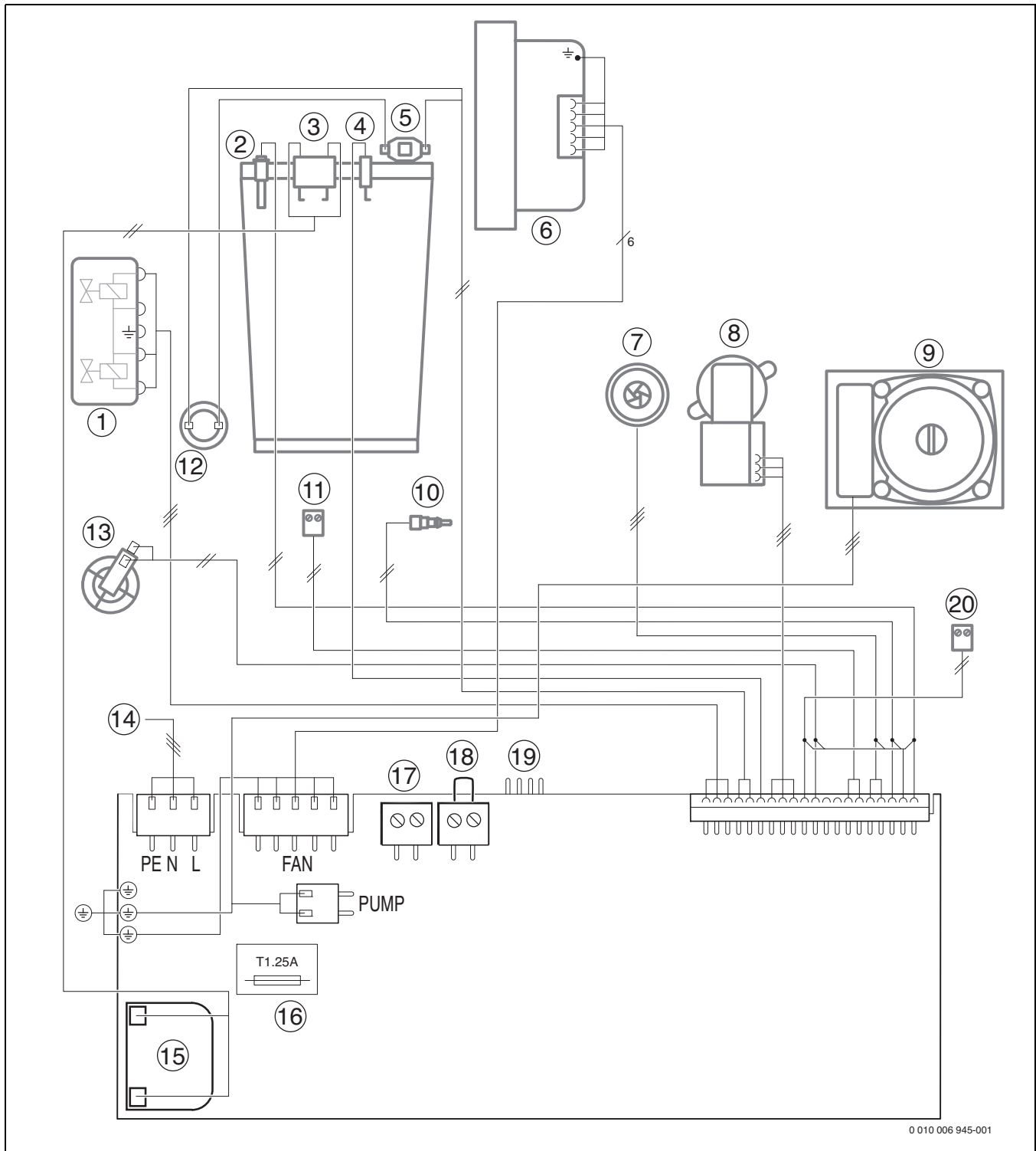
Res. 66 Elektrik hatları
