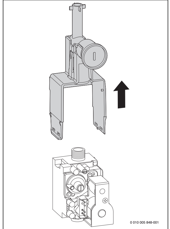
Res. 61 Gaz armatürünün sökülmesi, plastik dış mantonun çıkarılması
