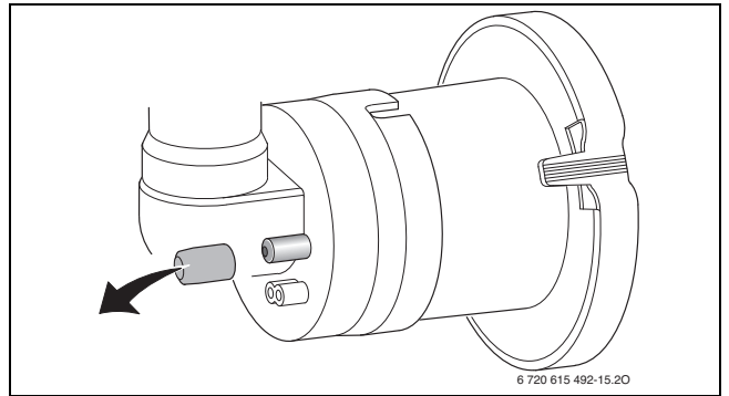
Res. 43 Karıştırma ünitesindeki ölçüm ağızı
