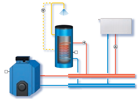
Funzione base dell'apparecchio di regolazione Logamatic 4211 impiegato con una caldaia a basamento
