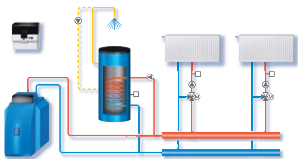
Funzione base dell'apparecchio di regolazione Logamatic 4121 impiegato con una caldaia a basement EMS, due circuiti riscaldamento e la produzione di acqua calda
