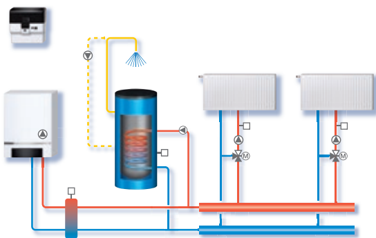
Funzione base dell'apparecchio di regolazione Logamatic 4121 impiegato con una caldaia murale EMS, due circuiti riscaldamento e la produzione di acqua calda
