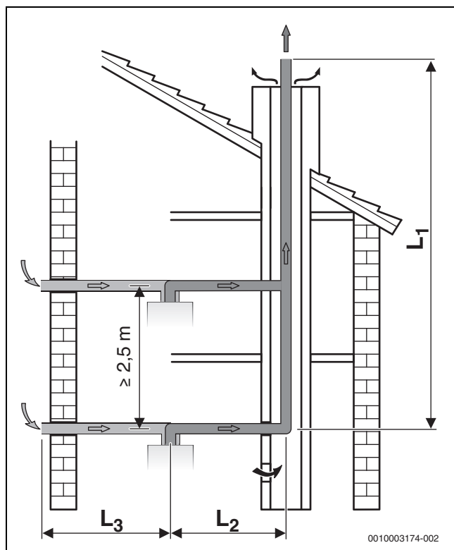
Рис. 18 Подключение нескольких котлов с раздельными трубами по C 83(x)
