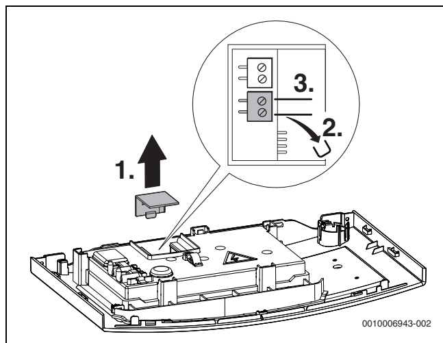
Рис. 27 Подключение регулятора
