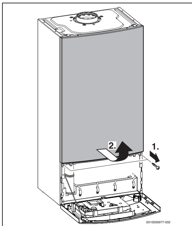
Рис. 24 Снятие передней облицовки
