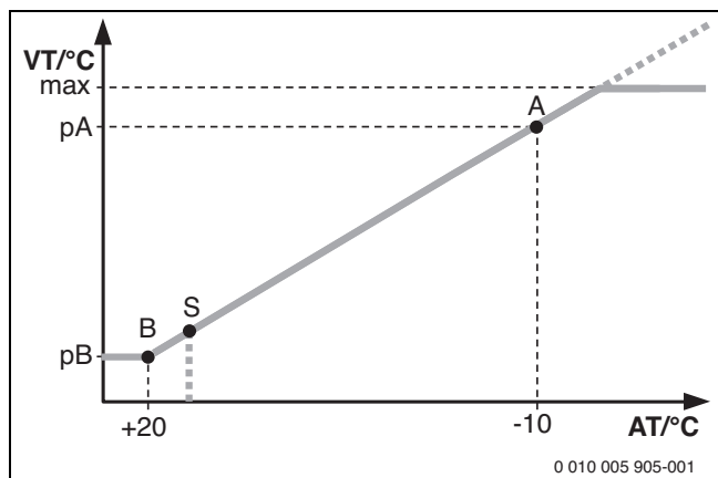
Рис. 67 Отопительная кривая
