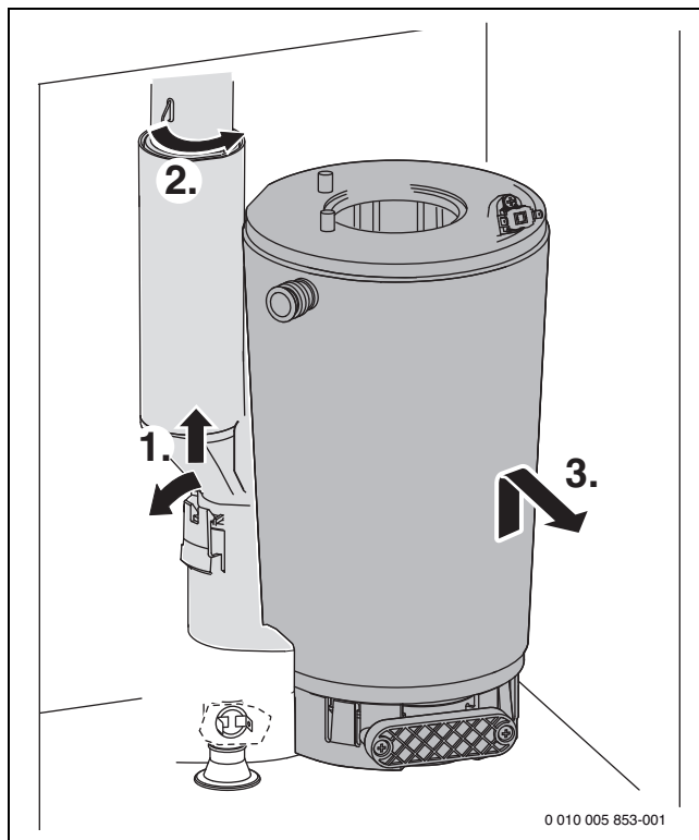
Рис. 65 Демонтаж теплообменника
