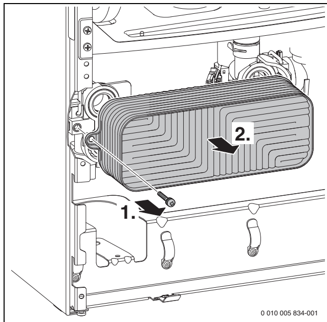
Рис. 57 Демонтаж пластинчатого теплообменника
