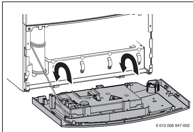
Рис. 23 Установите блок управления в положение для обслуживания
