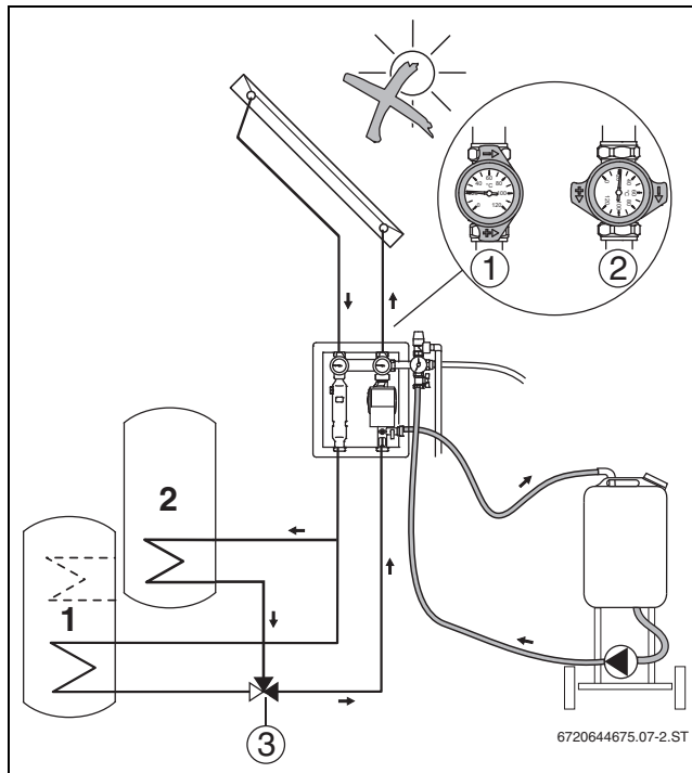
Рис. 30 Промывка бака 2
