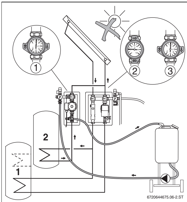
Рис. 29 Промывка бака 2
