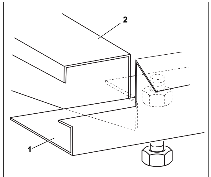
Şekil 39 Uzunlamasına rayın çapraz traverseye yerleştirilmesi
