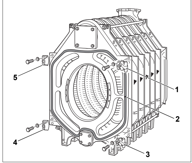
Şekil 31 Menteşe kancalarının ve kapama çıtalarının montajı
