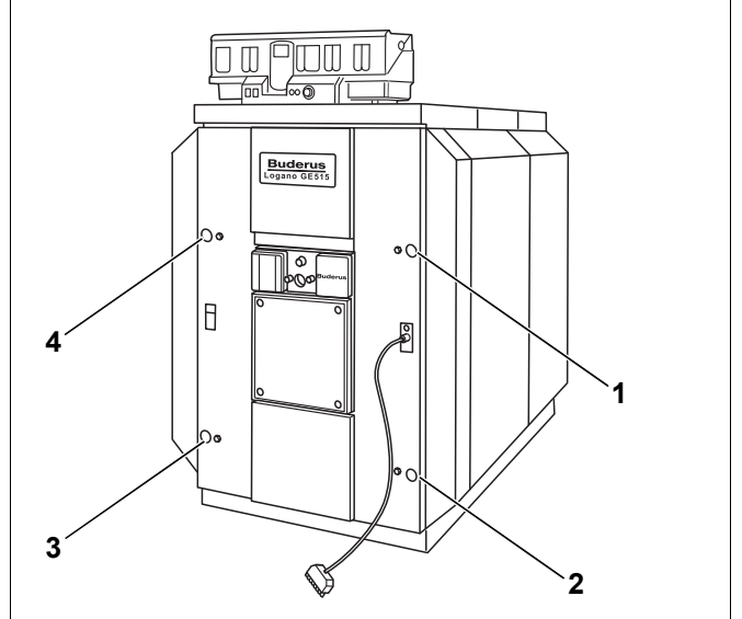
Şekil 71 Brülör kapağı bağlantı yerleri
