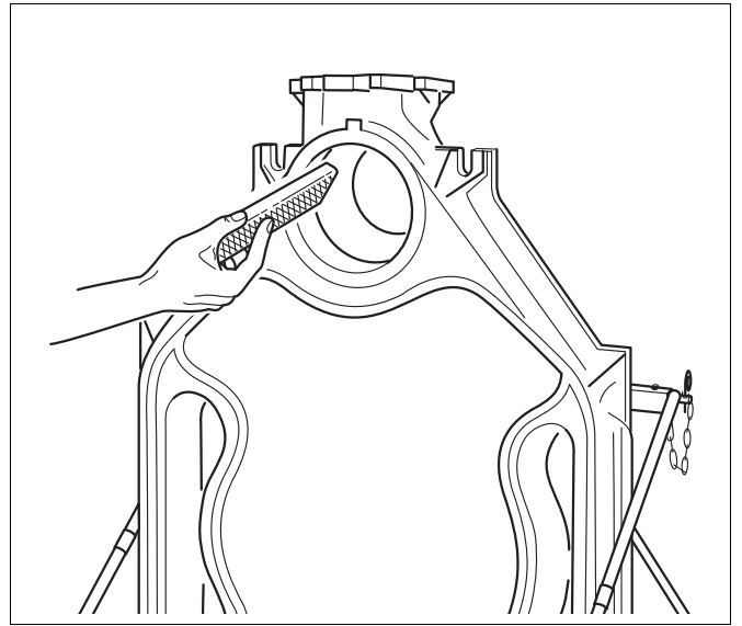
Şekil 12 Çapakların temizlenmesi
