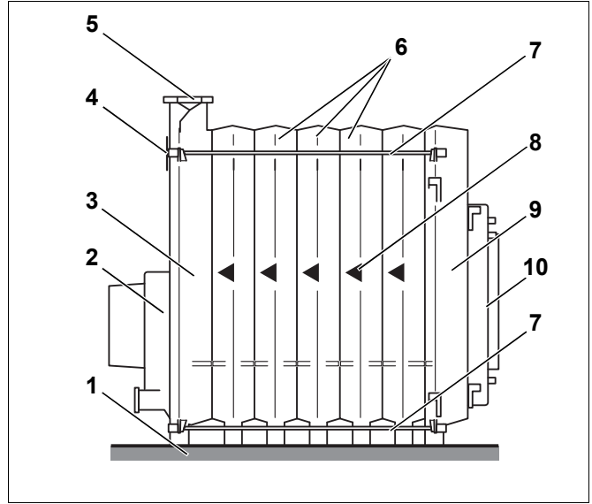
Şekil 8 Kazan bloğu
