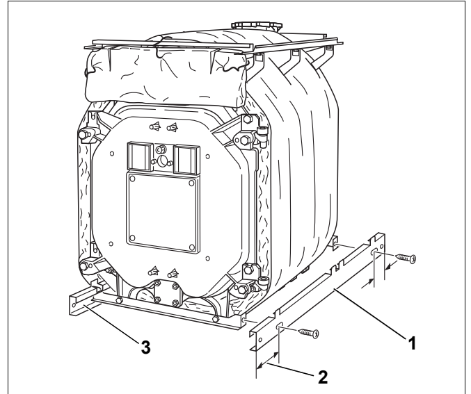
Şekil 47 Yan kaide raylarının montajı
