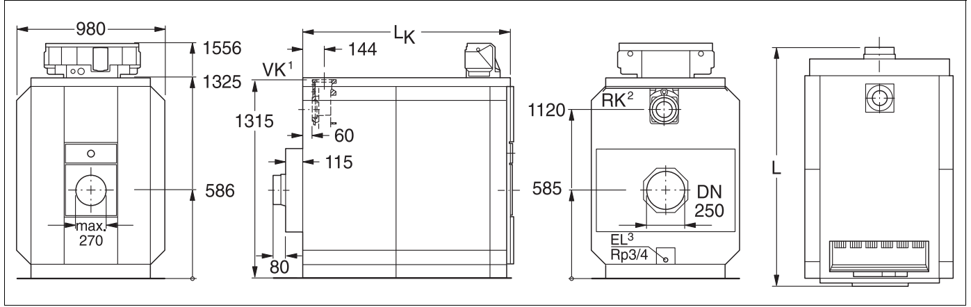
Şekil 3 Logano GE515 için teknik bilgiler (ölçüler mm)
