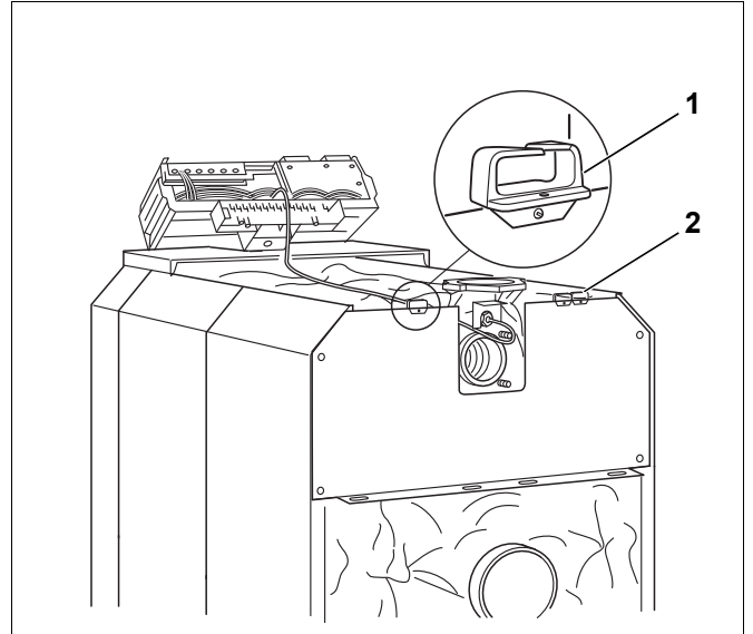
Şekil 63 Elektrik Bağlantısı
