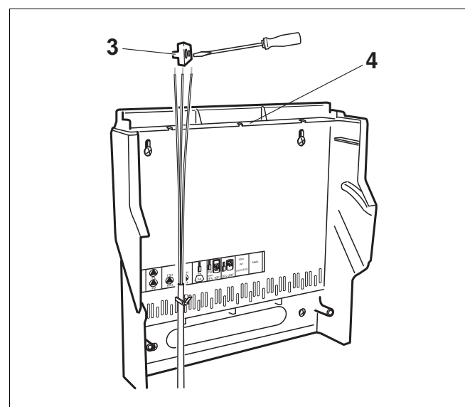
Рис. 6 Крепление проводов
