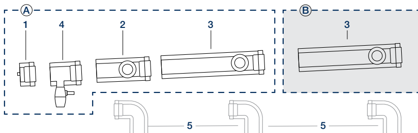
2-й вариант - с вводом в коллектор сбоку
