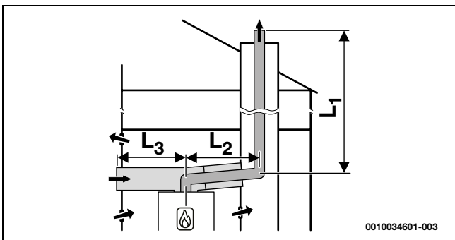
C93x Misto intubato a tetto
