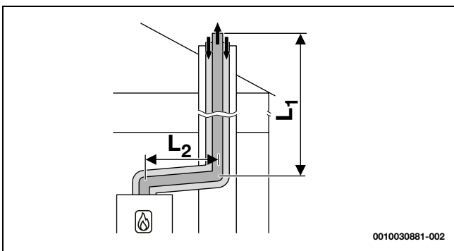
C53 Sdoppiato nel cavedio
