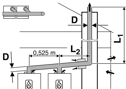
Lunghezze equivalenti massime ammesse per sistemi modulari di caldaie Logamax plus GB272, in PRESSIONE NEGATIVA, con collettori di scarico fumi in PPTl rigido, tipo B23p, in linea TL
