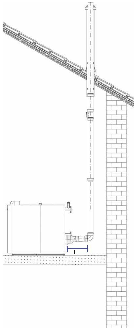
Variante 3 Centrale termica sotto tetto
