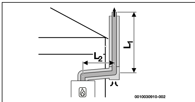
B52/B23p Misto intubato a tetto con aspirazione aria dal locale
