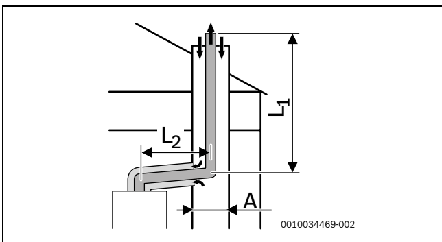
C93x Misto intubato a tetto
