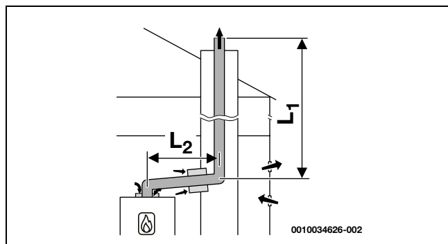
B52/B23p Misto intubato a tetto con aspirazione aria dal locale
