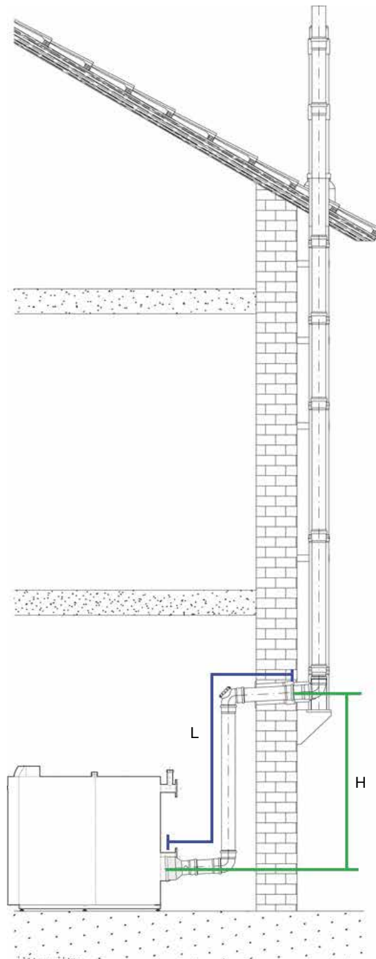
Variante 4 Sistema di parete esterna
