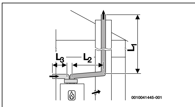
C53 Sdoppiato verticale in facciata
