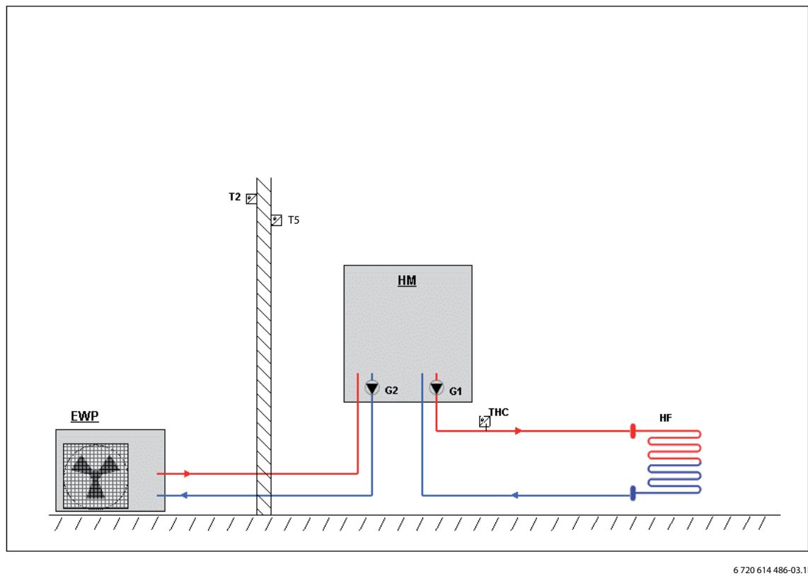
Fig. 2 Pompa di calore, modulo AWE e riscaldamento a pavimento
