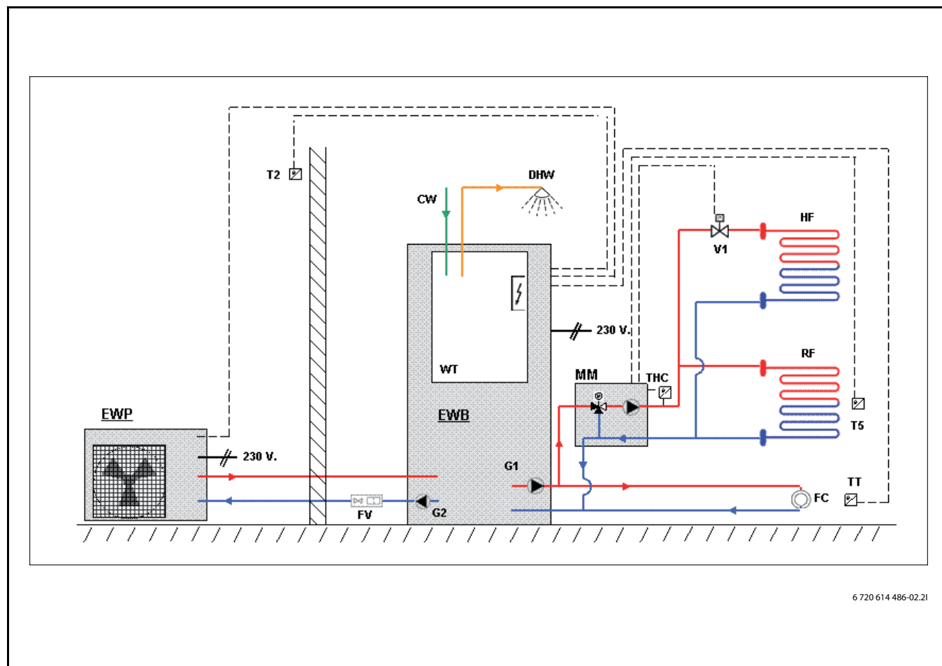
Fig. 1 Pompa di calore, modulo AW con accumulatore produttore di acqua calda integrato e riscaldamento a pavimento
