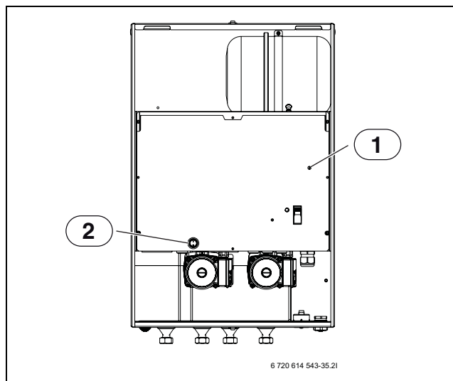
Fig. 30 Modulo idraulico interno AW (AWE)
