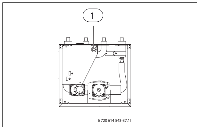
Fig. 28 Modulo miscelatore
