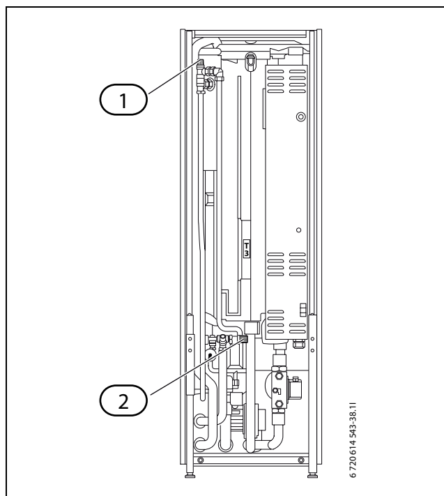
Fig. 25 Modulo AW (AW E9T)
