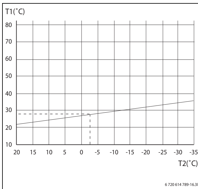
Fig. 9 Curva di riscaldamento, esempio di curva per impianto di riscaldamento a pavimento
