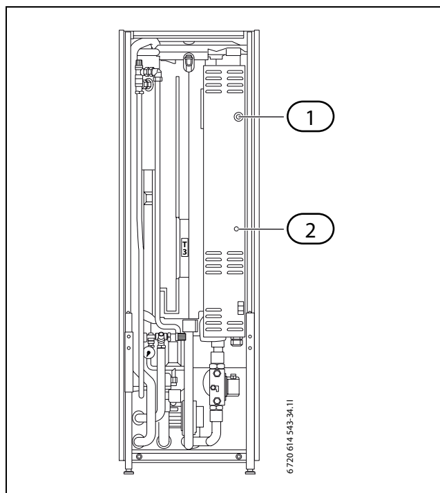
Fig. 29 Modulo idraulico interno AW (AW 9T)
