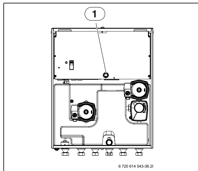
Fig. 27 Modulo idraulico interno AW (AW B9)
