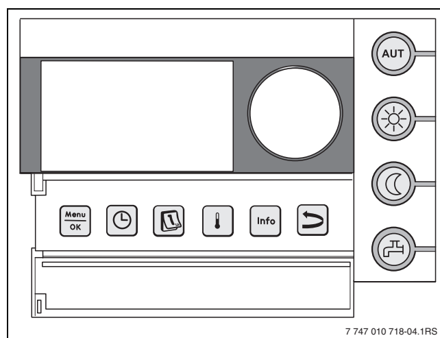
Fig. 8 Unità di servizio (ad es. RC35, con sportellino aperto)
