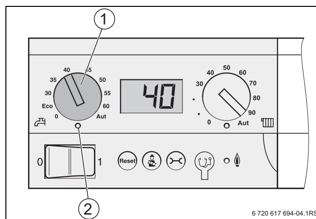
Fig. 3 Manopola valore nominale acqua calda sanitaria
