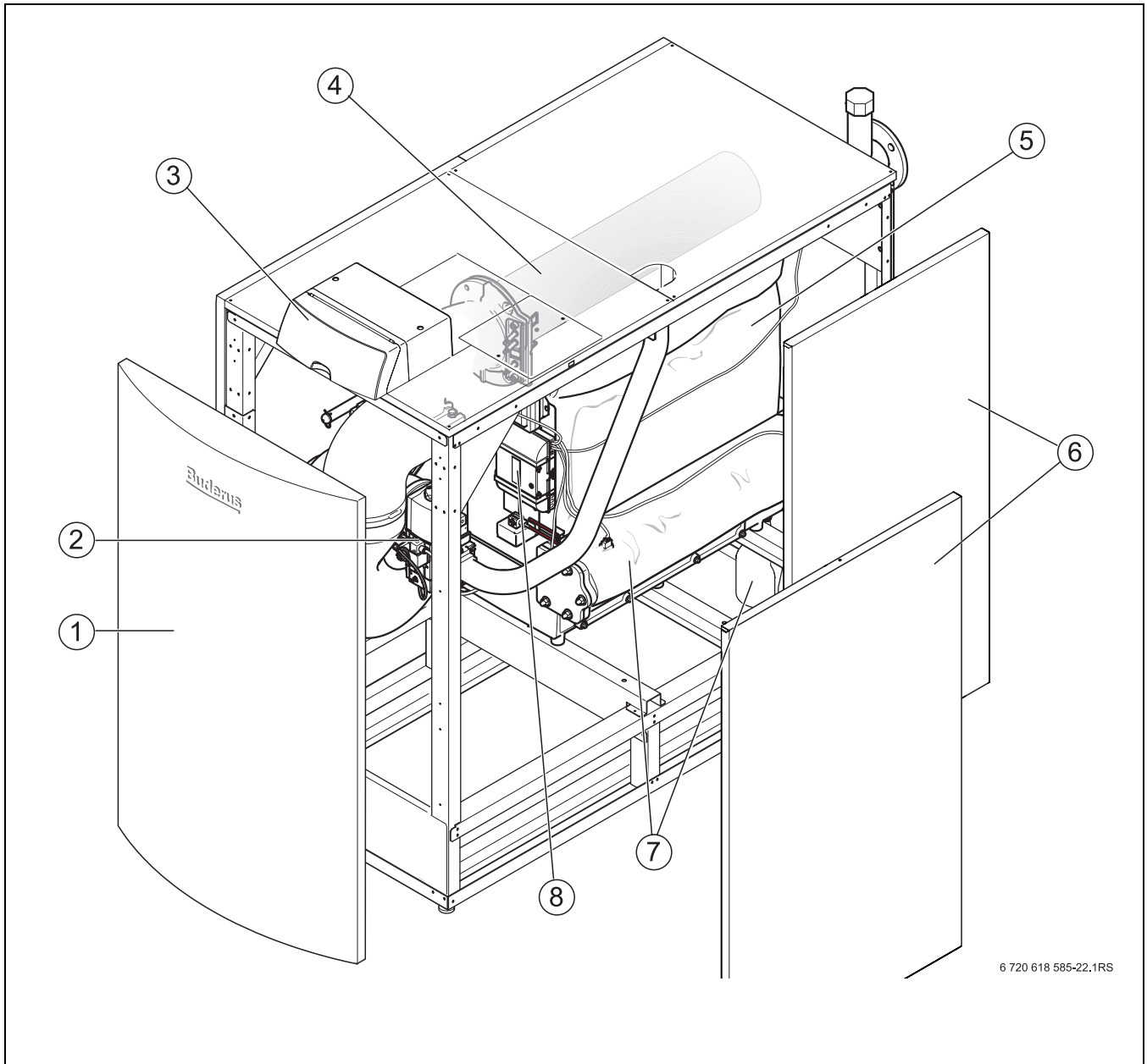
Fig. 1 Componenti principali della Logano plus GB402
