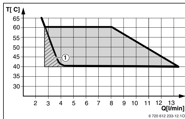
Fig. 9 Diagramma per una temperatura di ingresso dell'acqua fredda di +15°C
