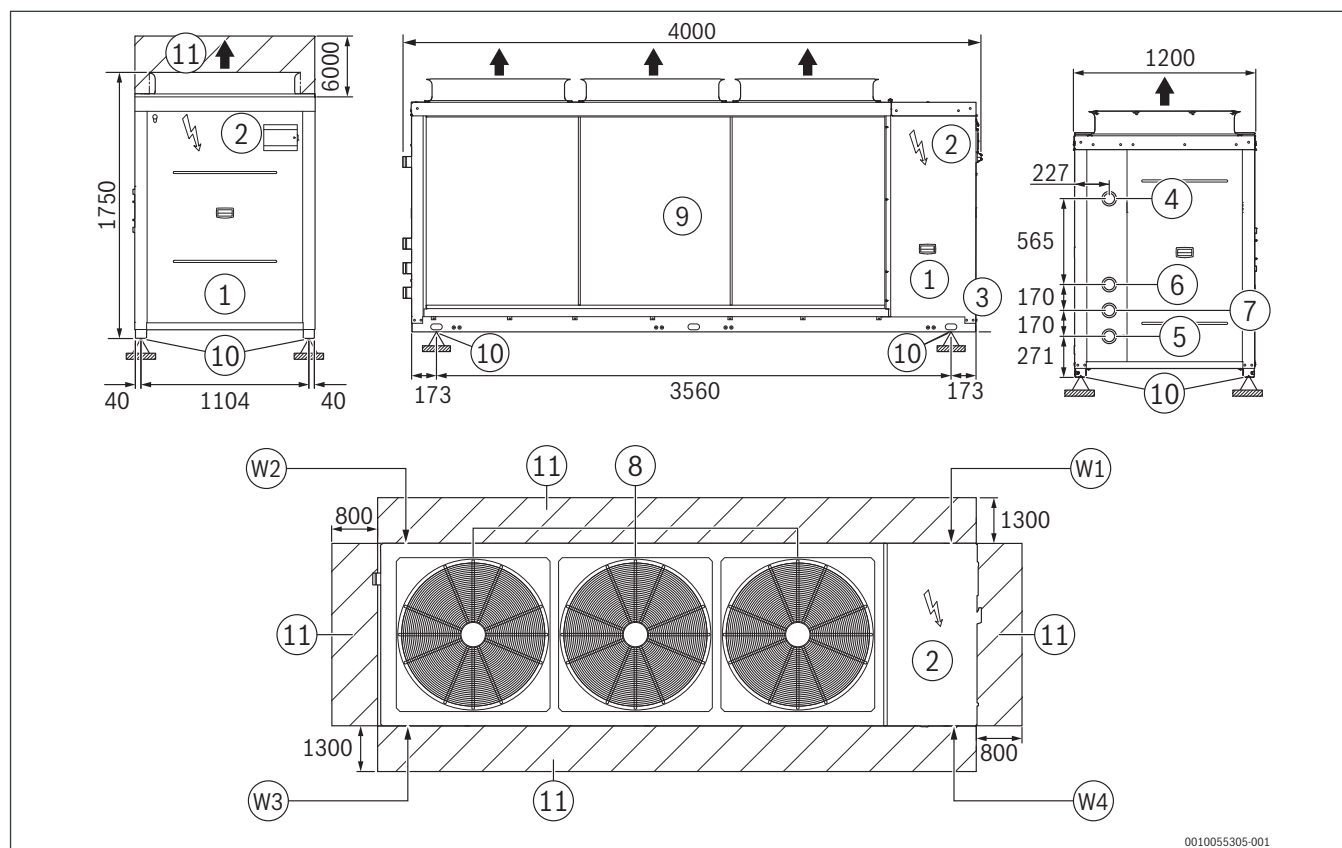
obr. 30 Rozměry WLW276-65, WLW276-75 a WLW276-89 (mm)
